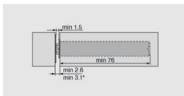
Pletina para empotrar para cierre TOCA-TOCA.
